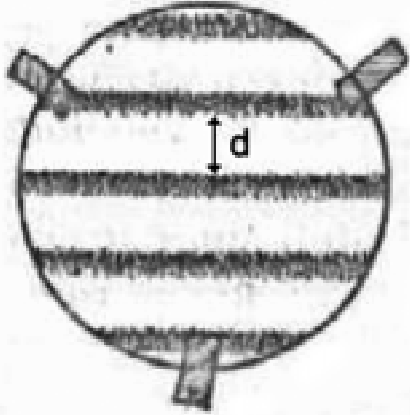
Figura 8. a) Superficie esférica convexa
