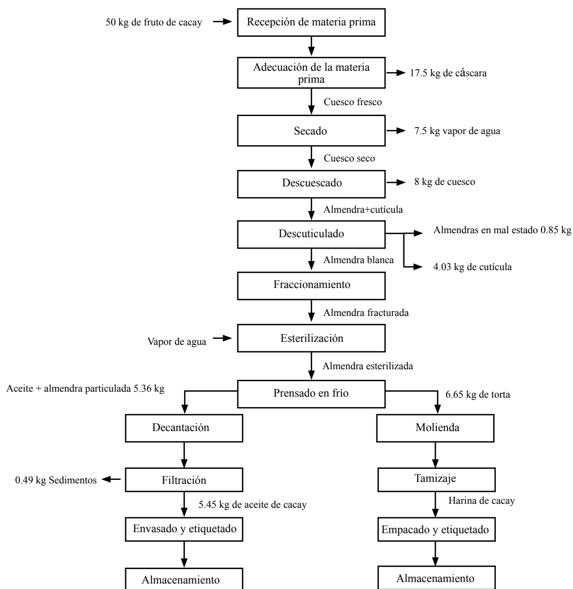
Figura 2. Diagrama de proceso y balance de materia de la extracción del aceite de cacay
