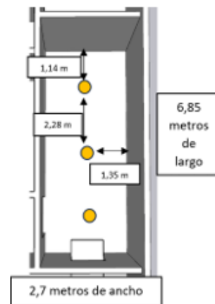
Figura 6. Distribución de las luminarias en el área de adecuación de materia prima
