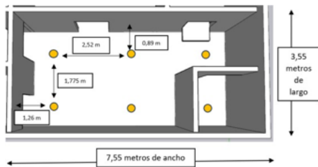
Figura 5. Distribución de las luminarias 1 en el área de proceso
